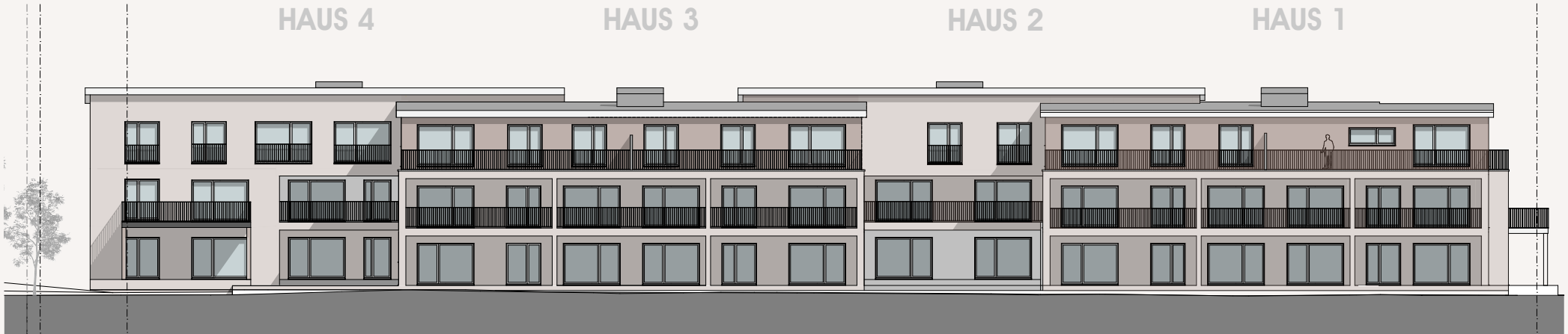
LINKE SEITENANSICHT . ANSICHT WEST
