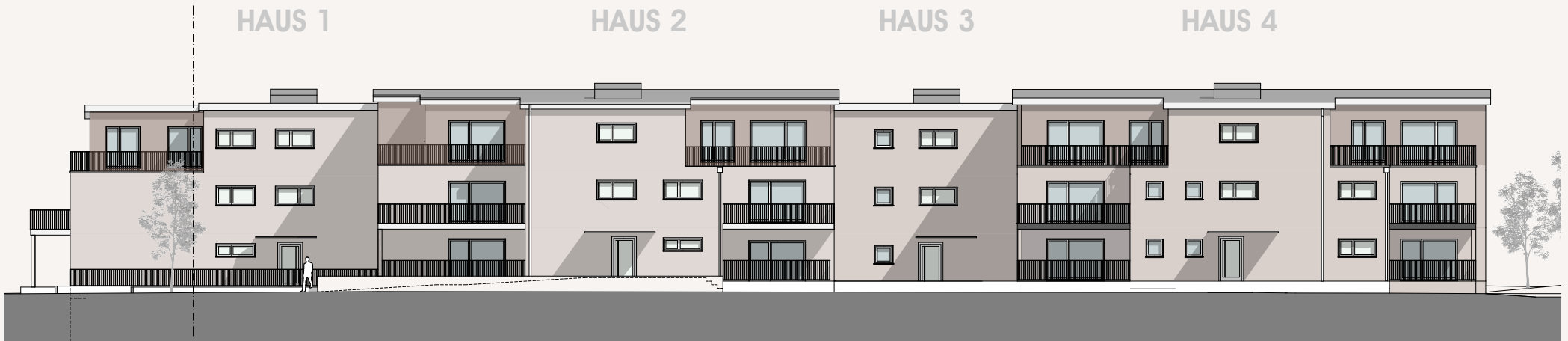
RECHTE SEITENANSICHT . ANSICHT OST
