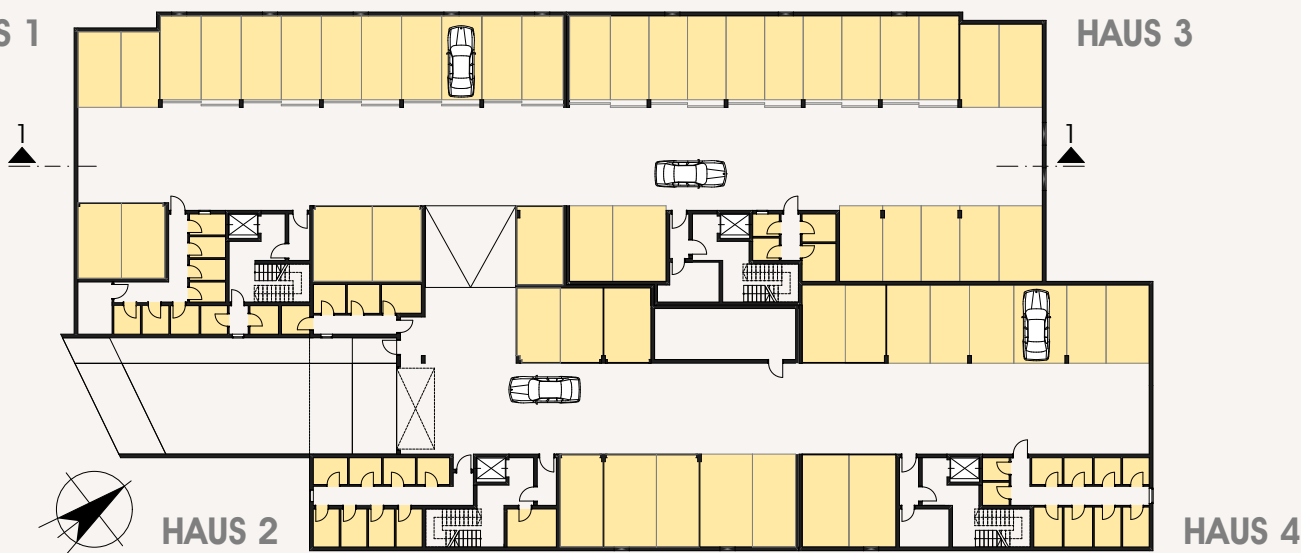
ÜBERSICHTSPLAN . GRUNDRISS UNTERGESCHOSS
