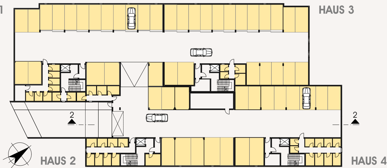
ÜBERSICHTSPLAN . GRUNDRISS UNTERGESCHOSS
